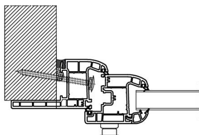
Remplissage panneau lisse
