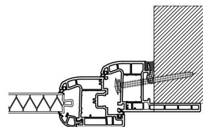
Remplissage panneau lambris
