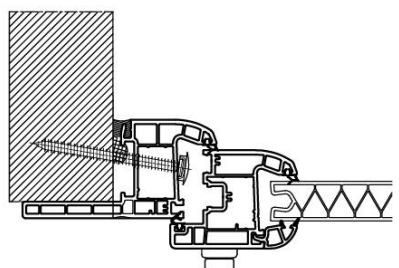
Remplissage panneau lambris
